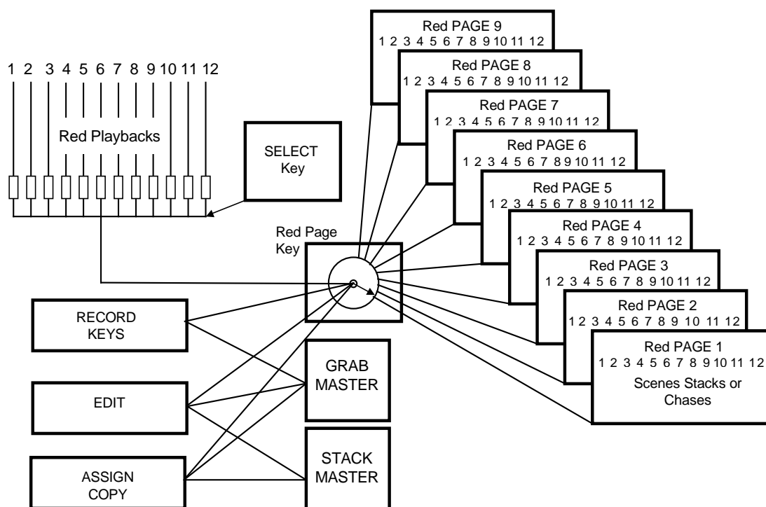
Maxim S : structure de mémoire de base.
